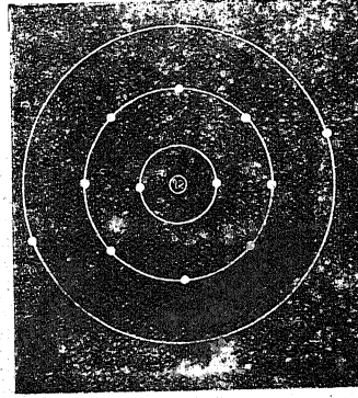
चित्र १३५—मगनीसियम परमाणु का कल्पित चित्र जिसके बीच में धनाणु है जिसकी विजली की मात्रा १२ है। चारों ओर बारह ऋणाणु चकर लगाने हैं।
